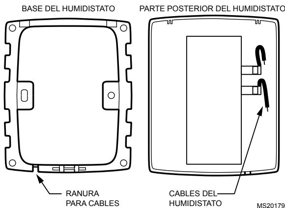
Fig. 11. Base del humidistato y vista posterior.
